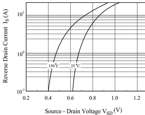
I_S - V_{SD}
